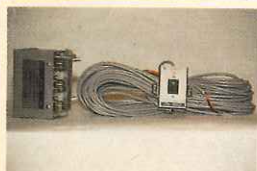
CORONA CX-1000 190.- «N-Anschluss» Antennen-Umschalter für Dachmontage (bis 1300 MHz). Best.-Nr. 504-910
