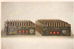
ZETAGI B-300/B-550 PS 275.-/435.- KW-Leistungsverstärker, max. 200/300 (400/600SSB) W. Best.-Nr. 575-300/575-550 Für CB-Funk nicht gestattet!
